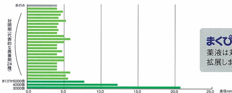
図1. プラスチックシート上における各薬液の滴下30秒後の広がり(直径mm) 石原産業中央研究所内
