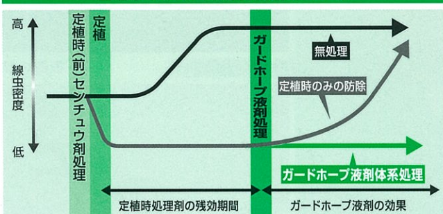
土壌中のセンチュウ密度の推移モデル
